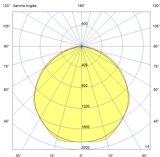
Curba de distribuție a intensității luminoase [Cd/1000lm]
