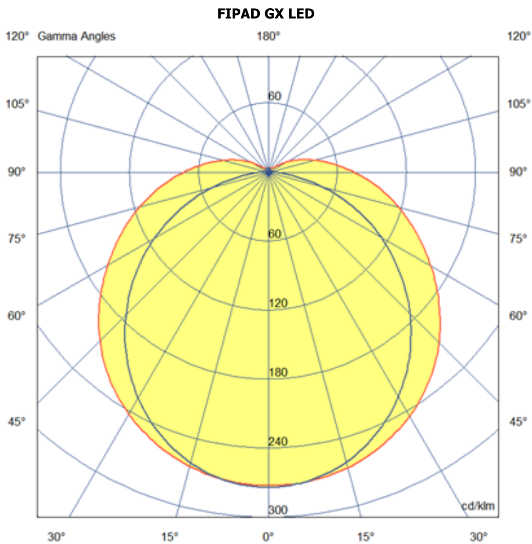
Curba de distribuție a intensității luminoase [ \text{Cd}/1000\text{lm} ]
